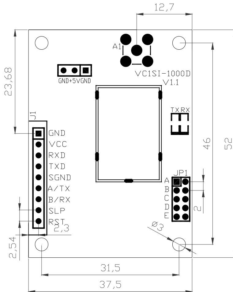
图 2.产品尺寸图
