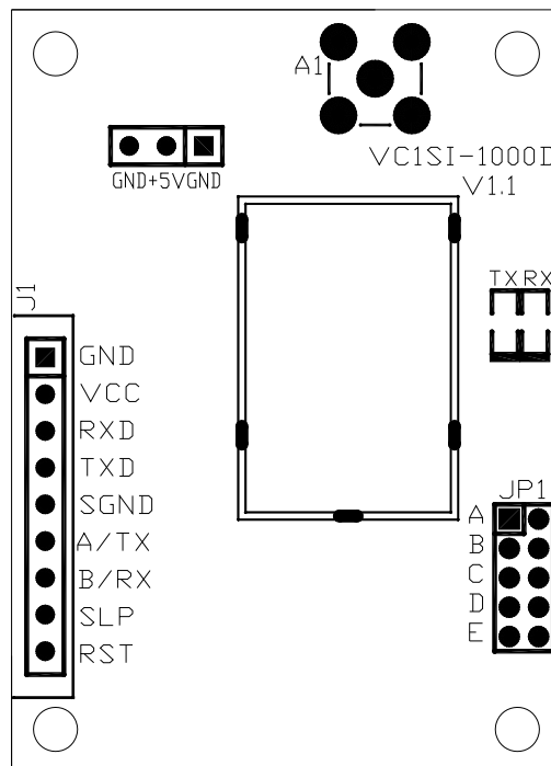
图 1.引脚位置图
